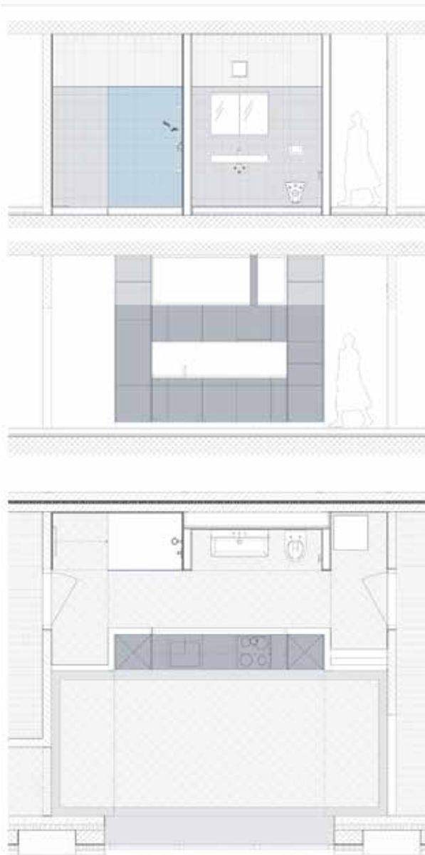
Ansichten Bad und Küche OG
