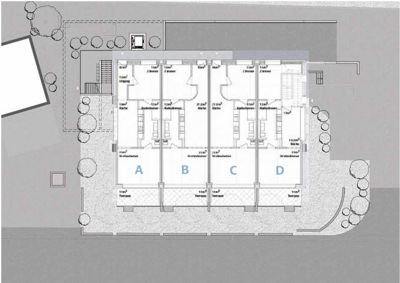
Grundriss EG
